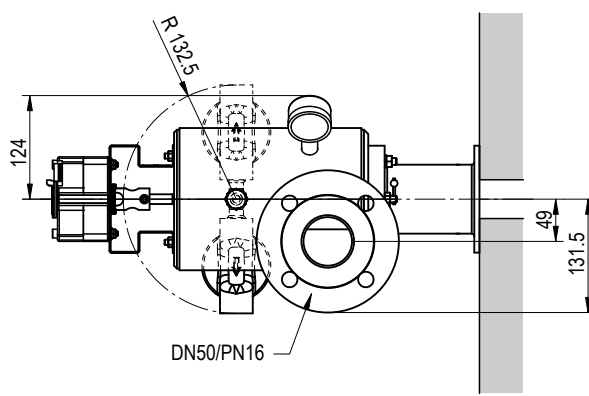
FELÜLNÉZET
