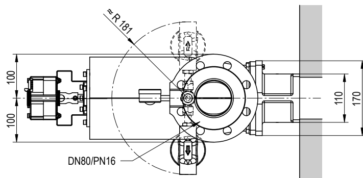
FELÜLNÉZET
