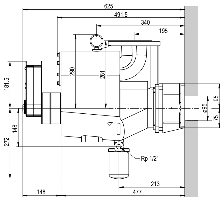
FELÜLNÉZET
