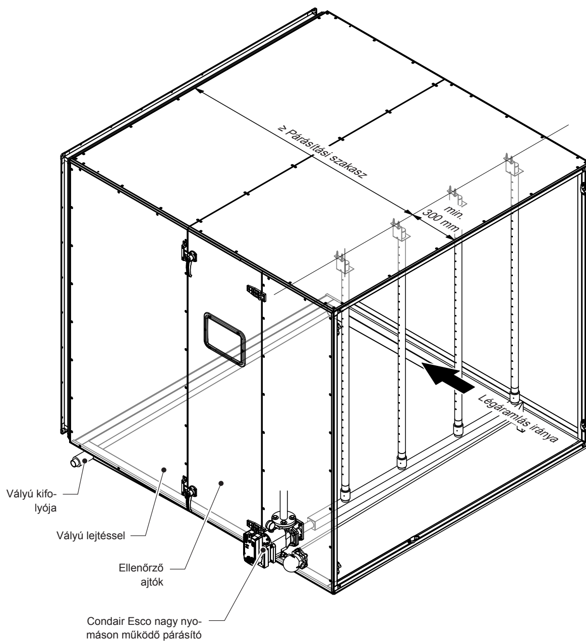
Ábr. 28: DR73 csatorna/szellőztetőberendezés / az elé-/utánkapcsolt akadályoktól való távolság
