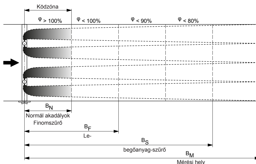
Ábr. 29: A párasítási szakaszok terminológiája
