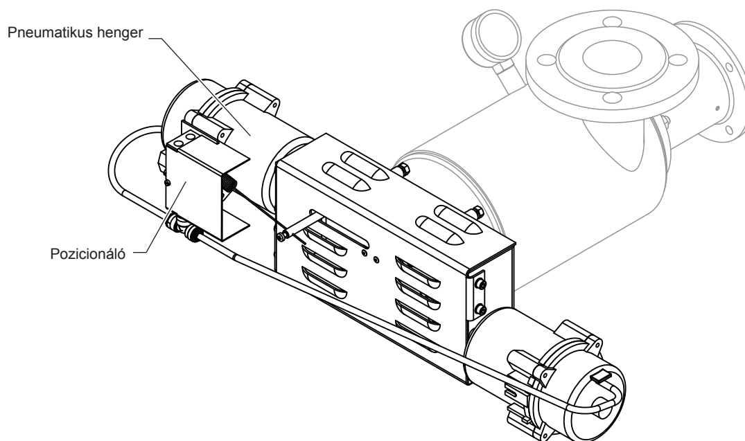
Ábr. 18: A Sauter AK41 pneumatikus hajtás és a Sauter XSP31 pozicionáló
