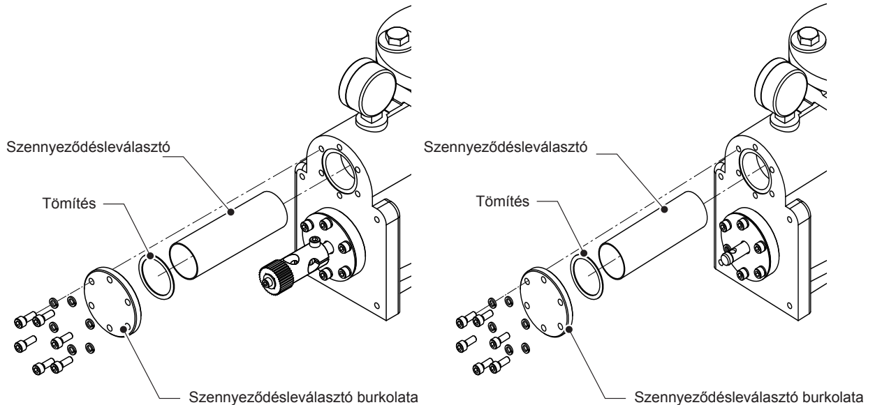
Ábr. 55: A szennyeződésleválasztó kiszerelése
