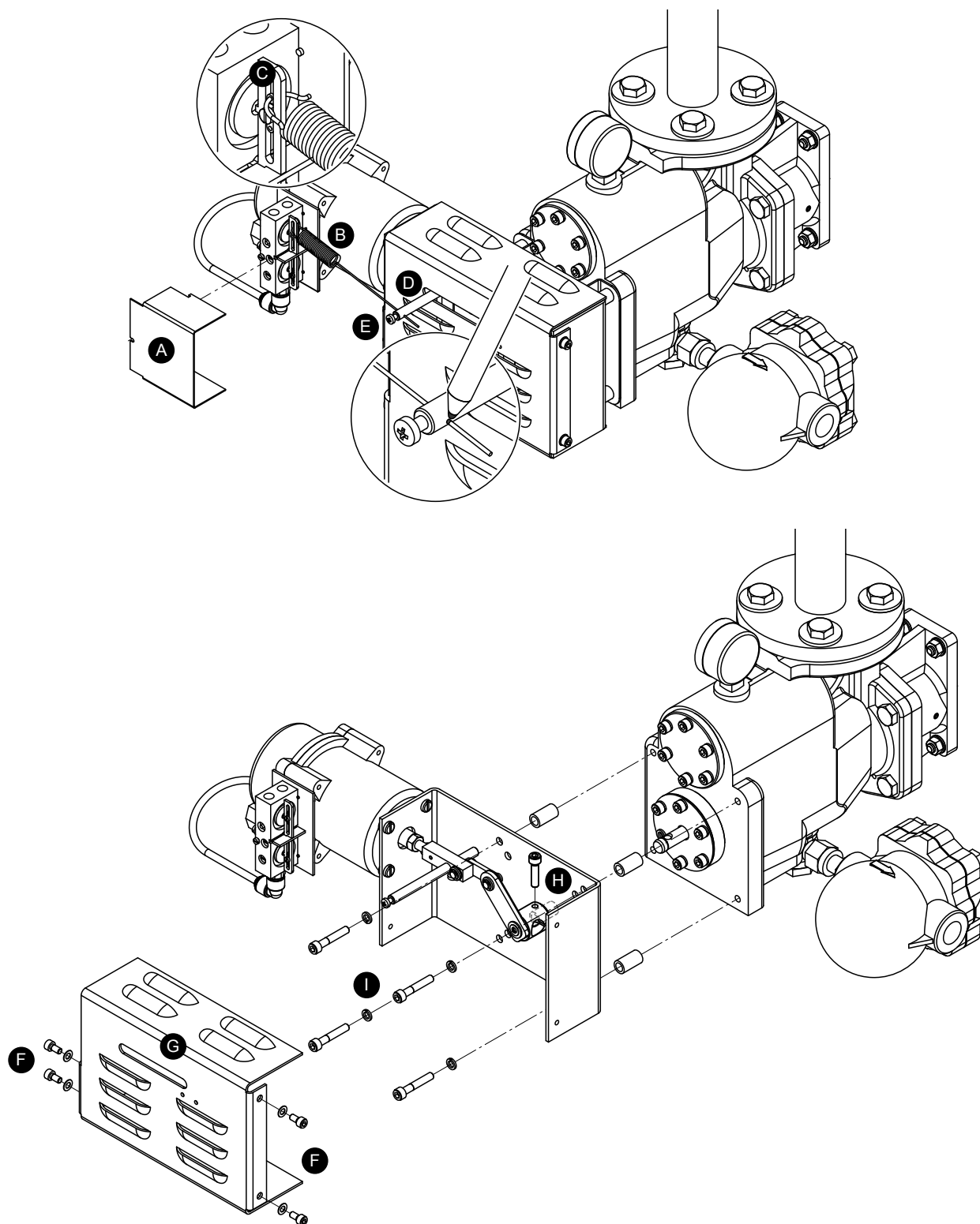
Ábr. 54: A pneumatikus hajtás kiszerezése
