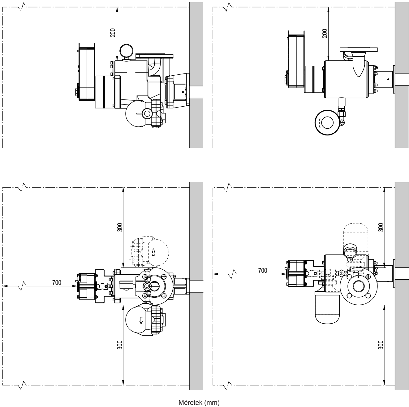
Ábr. 56: A szelepegység körül előírt szabad terek
