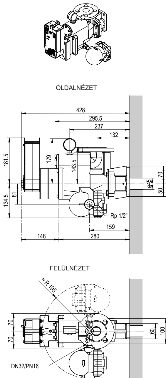
Ábr. 59: Méretrajz: Esco 10 (gömbgrafitos öntöttvas) úszógolyós kondenzedénnyel, CA150A-MP elektromos hajtással
