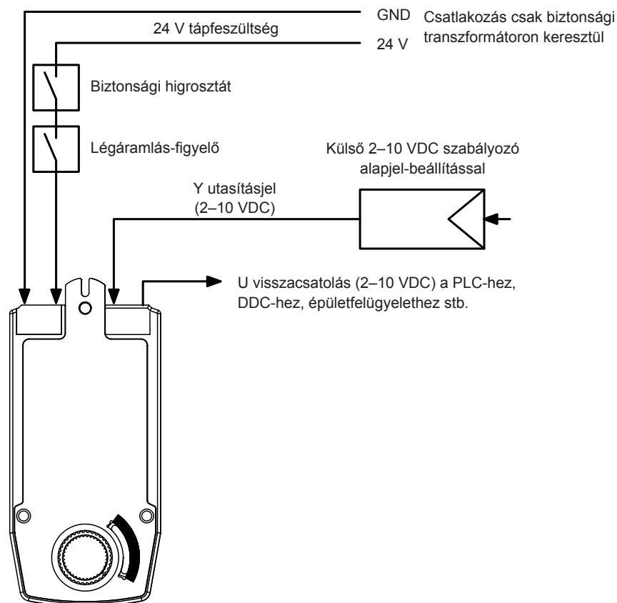
Ábr. 34: A CA150A-MP hajtás szabályozási sémája
