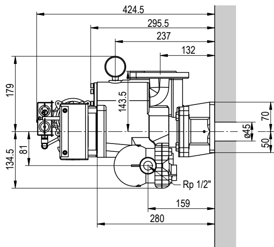
FELÜLNÉZET
