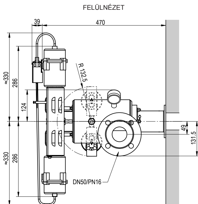
Ábr. 74: Méretrajz: Esco 20 (rozsdamentes acél) úszóharangos kondenzedénnyel, Sauter AK41 pneumatikus hajtással
