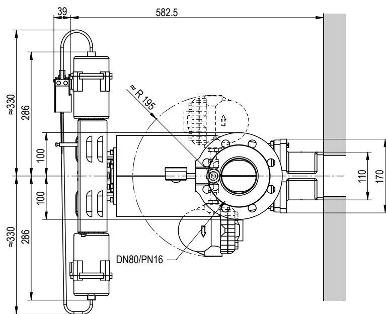
Méreték (mm)
