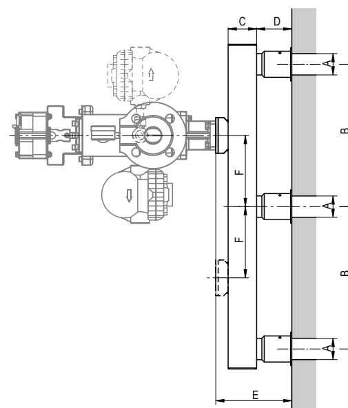
FELÜLNÉZET
