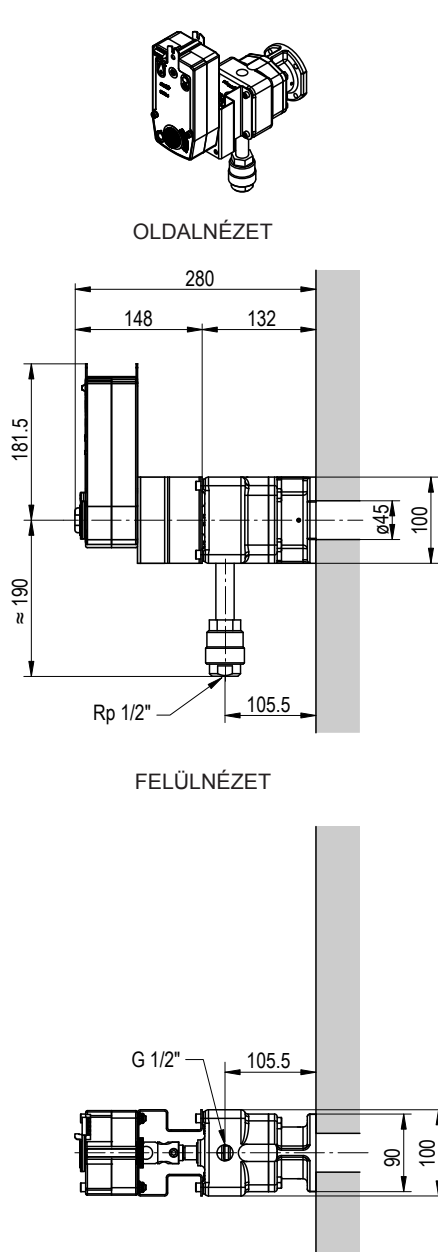
Ábr. 57: Méretrajz: Esco 5 (gömbgrafitos öntöttvas) CA150A-MP elektromos hajtással
