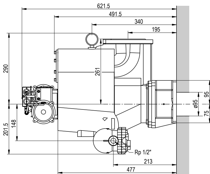
FELÜLNÉZET
