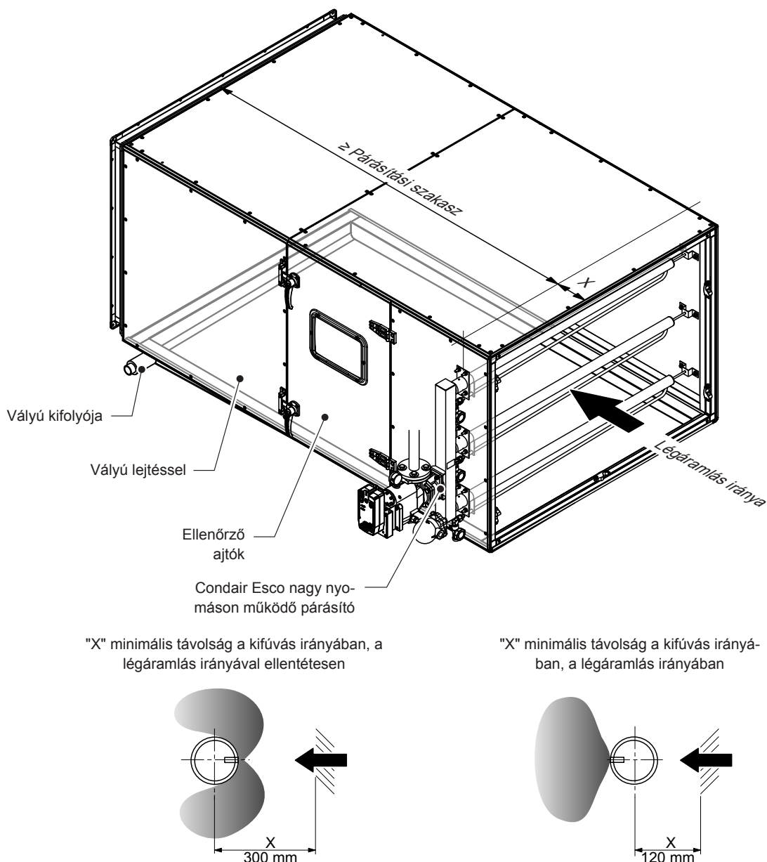
Ábr. 27: DL40 csatorna/szellőztetőberendezés / az elé-/utánkapcsolt akadályoktól való távolság
