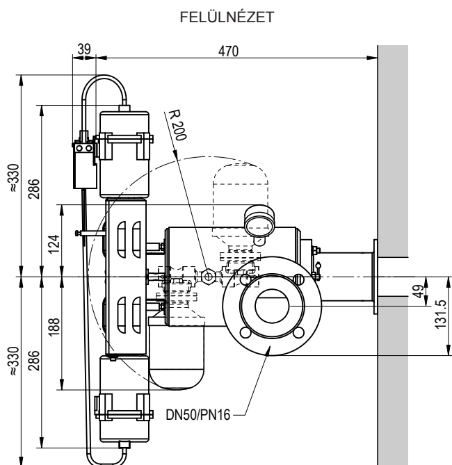
Ábr. 73: Méretrajz: Esco 20 (rozsdamentes acél) úszógolyós kondenzedénnyel, Sauter AK41 pneumatikus hajtással
