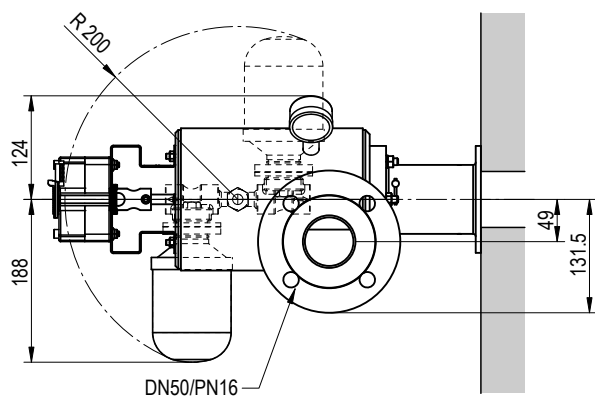
FELÜLNÉZET
