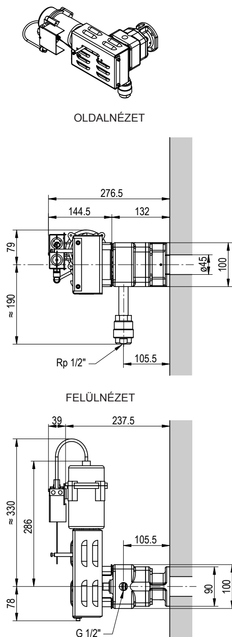
Ábr. 58: Méretrajz: Esco 5 (gömbgrafitos öntöttvas) Sauter AK41 pneumatikus hajtással
