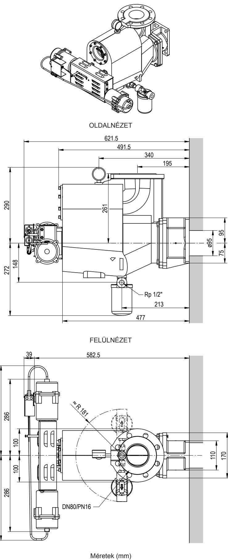
Ábr. 78: Méretrajz: Esco 30 (gömbgrafitos öntöttvas) úszóharangos kondenzedénnyel, Sauter AK41 pneumatikus hajtással
