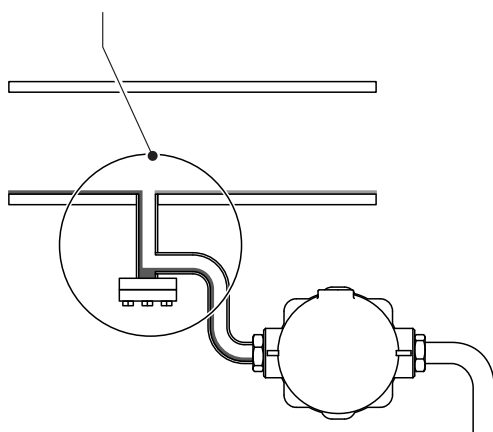
Ábr. 40: Hibás kondenzvíz-elvezetések
