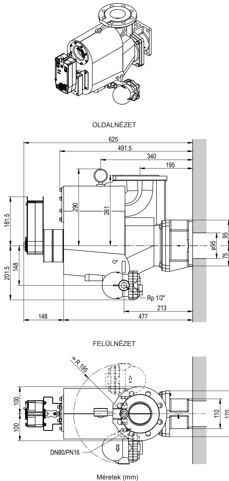
Ábr. 75: Méretrajz: Esco 30 (gömbgrafitos öntöttvas) úszógolyós kondenzedénnyel, CA150A-MP elektromos hajtással
