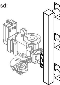
OLDALNÉZET
