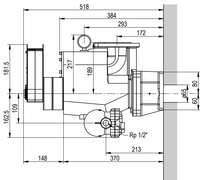
FELÜLNÉZET
