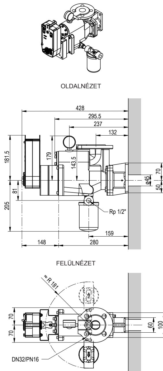
Ábr. 60: Méretrajz: Esco 10 (gömbgrafitos öntöttvas) úszóharangos kondenzedénnyel, CA150A-MP elektromos hajtással
