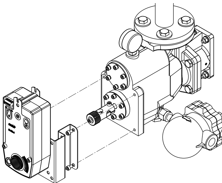
Ábr. 53: Az elektromos hajtás kiszerelése
