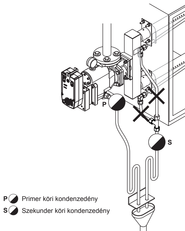
Ábr. 50: Nem megfelelően kivitelezett kondenzvíz-elvezető vezeték
