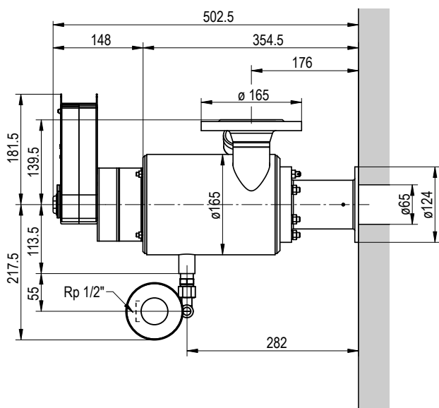
FELÜLNÉZET
