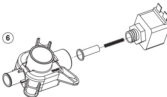
11. ábra: A leeresztőszelep szétszerelése
