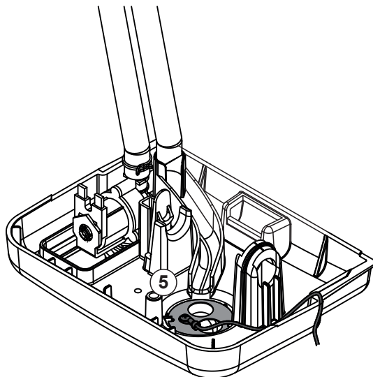
10. ábra: A földzárlat-megszakító kiszerelése
