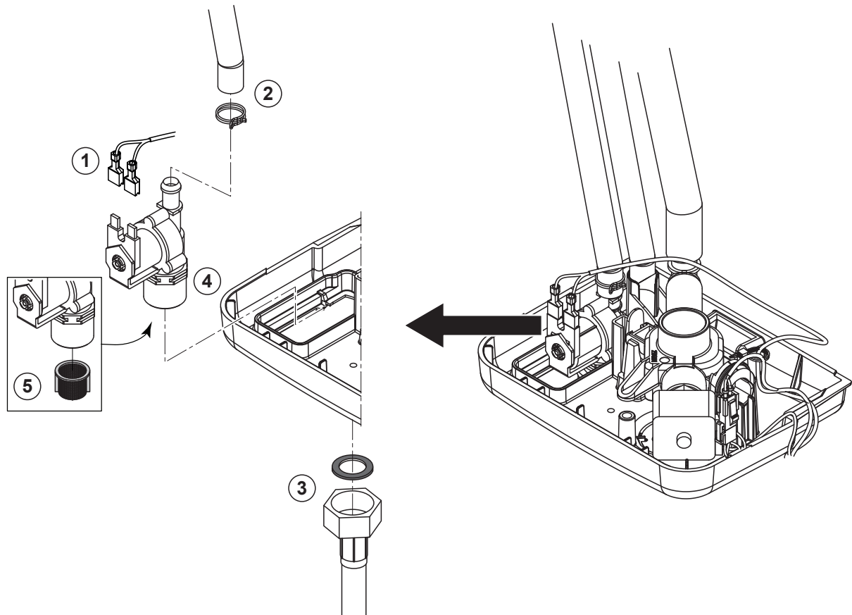
12. ábra: A szívószelep kiszerezése
